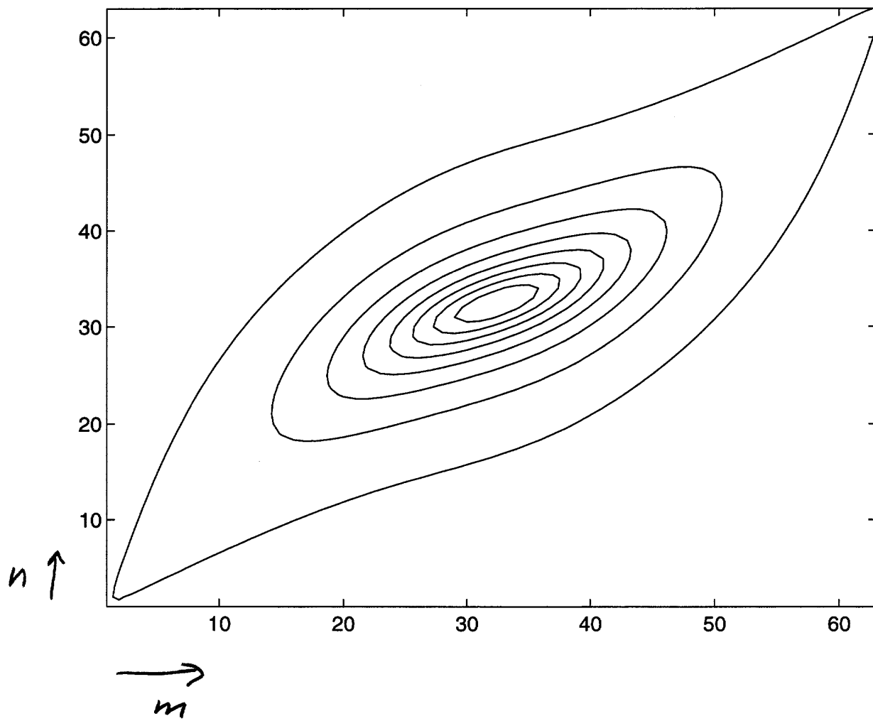
Contour Plot of MTF for (1 - 0.2 \cdot Z_1^{-1} - 0.2 \cdot Z_2^{-1} - 0.4 \cdot Z_1^{-1} \cdot Z_2^{-1})^{-1}
