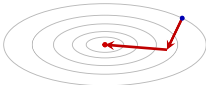
conjugate gradient
