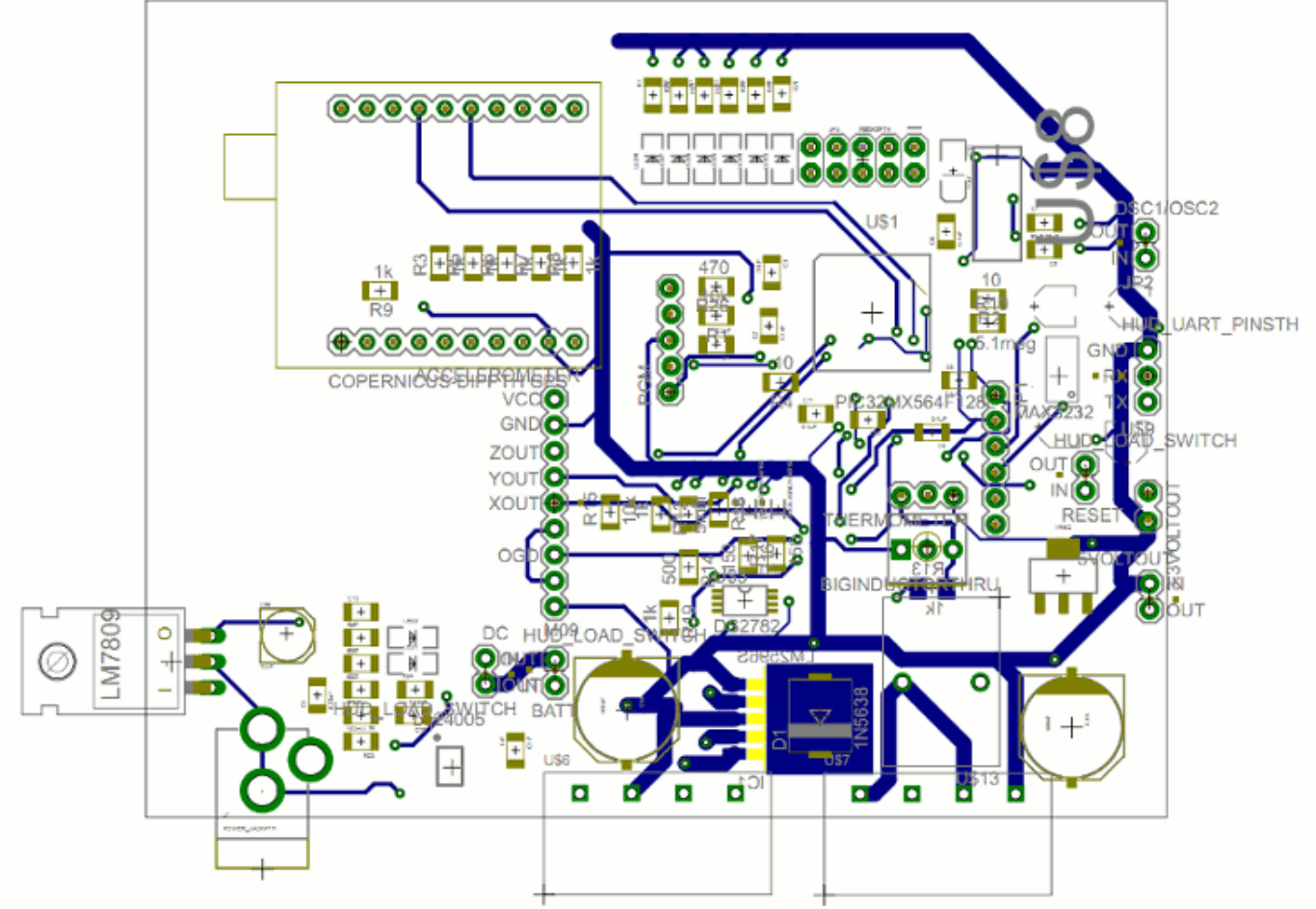
PCB - Bottom Layer
