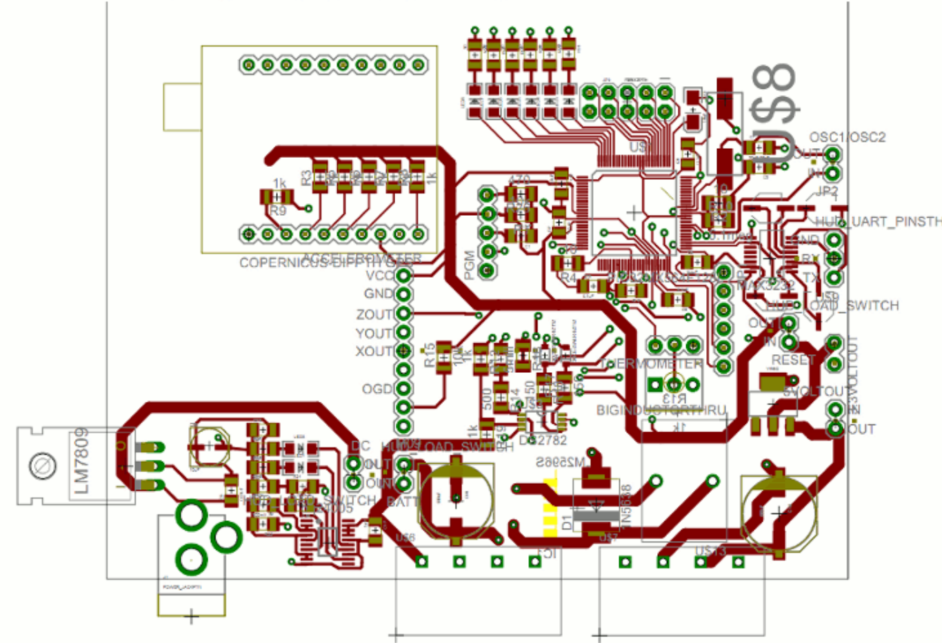
PCB - Top Layer
