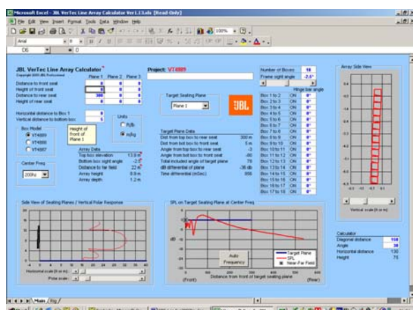
Fig 11. 18xVT4889 at 0deg splay angle, 200Hz. [-6dB@300m]
