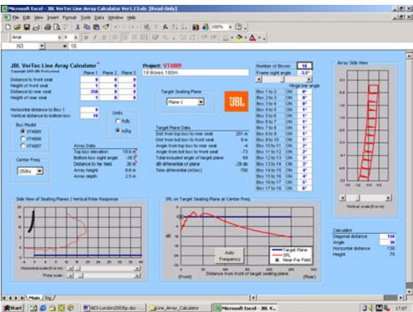
Fig A9. 18 Boxes 0,0,0,1,1,1,1,1,2,2,3,3,4,4,5,6 at 250Hz
