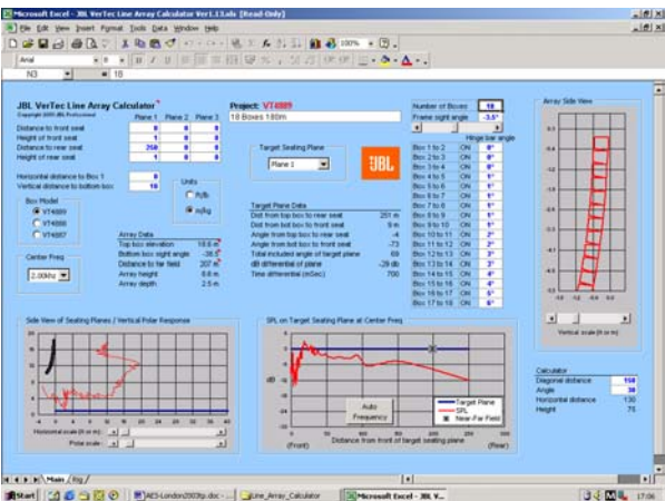
Fig A8. 18 Boxes 0,0,0,1,1,1,1,1,2,2,3,3,4,4,5,6 at 2kHz
