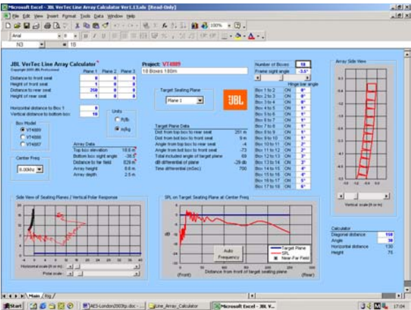
Fig A7. 18 Boxes 0,0,0,1,1,1,1,1,2,2,3,3,4,4,5,6 at 8kHz
